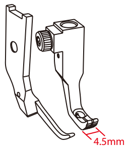
Presser foot width 外壓腳寬度: 6.5mm Feeding foot width 內壓腳寬度: 4.5mm
