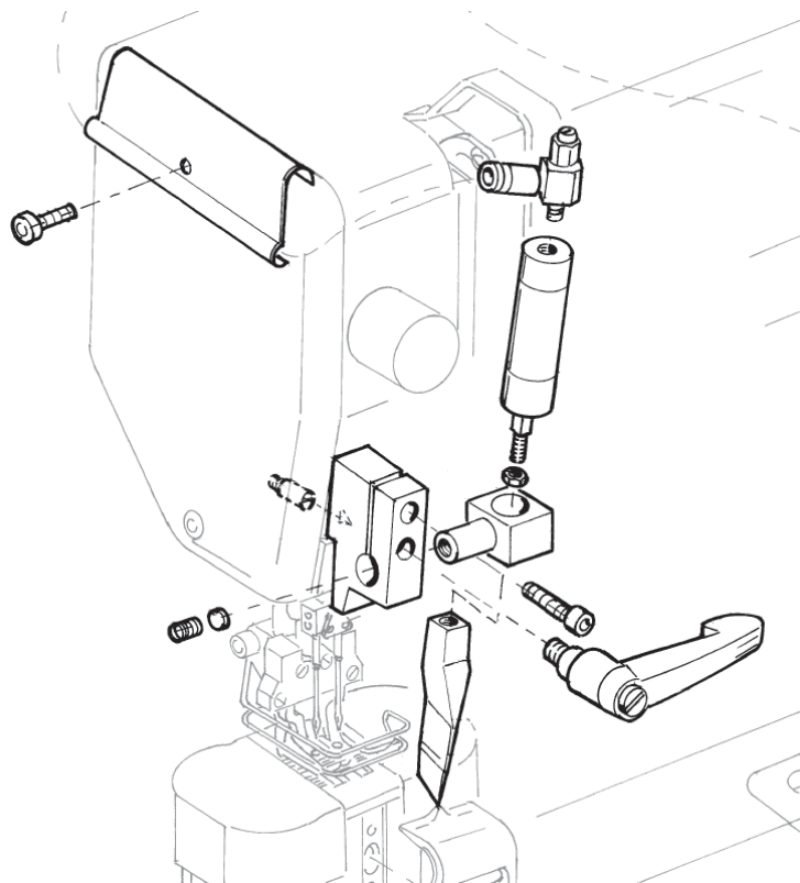
Pneumatic guiding set for 768 768 氣動傍位
