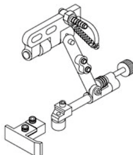
Long straight guide & 14mm dia. roller guide 長直形傍位及14mm直徑滾輪傍位
