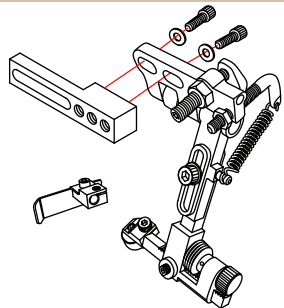
Long straight guide & 14mm dia. roller guide 長直形傍位及14mm直徑滾輪傍位 For most Pfaff machine models 適合大部份百福機種
