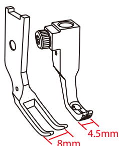
Presser foot width 外壓腳寬度: 8mm Feeding foot width 內壓腳寬度: 4.5mm
