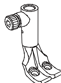
Feeding foot for center guide 中分刀雙針內壓腳
