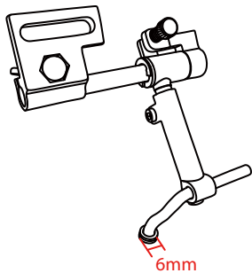
Roller guide 滾輪傍位: 6mm
