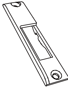
Needle plate for binding (Moving arm KH867) 包邊用針板 (配搭KH867擺架使用)
