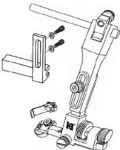
For Juki DU-141 重機DU-141用
