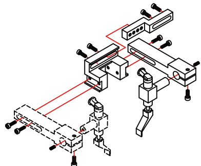
Pneumatic guide for universal machines 泛用型氣動傍位
