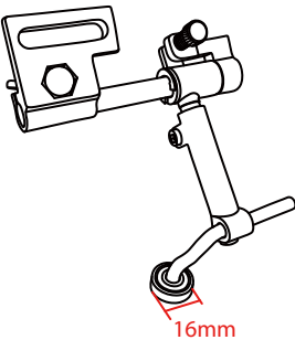
Roller guide 滾輪傍位 : 16mm
