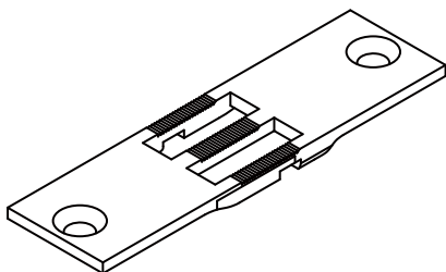
Needle plate for 867 867針板
