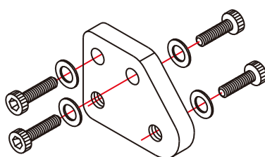
Bracket for Durkopp Adler 669, 867, 868 杜克普 669, 867, 868 用轉接配件
