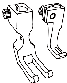
Regular foot 標準壓腳
