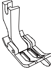
Right guide foot 右傍邊壓腳 Guiding distance 傍邊距離: 1.8mm
