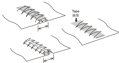
坑闊 Groove size: 4, 5, 6mm
