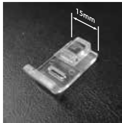
壓腳寬度 Presser foot width: 15mm 針孔寬度 Needle hole width: 8mm
