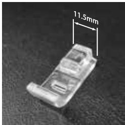
壓腳寬度 Presser foot width: 11.5mm 針孔寬度 Needle hole width: 6mm
