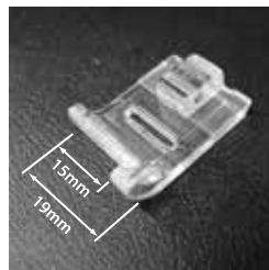
右傍邊壓腳 Right edge guiding foot
