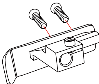
Zipper / Long straight guide (Dual functions) 拉鏈/直線兩用傍位
