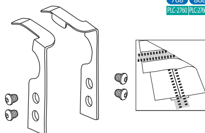
Downturn hemmer attachment 下摺邊助縫配件
