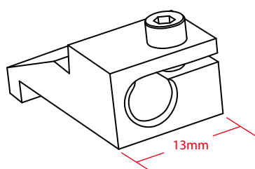
Zipper guide 拉鏈傍位
