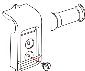
Belt guide 導帶器
