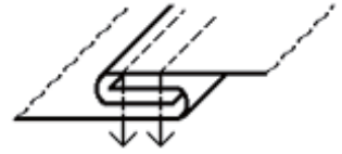
KHF 32 Side Seam Lapper (Japanese Style) 邊縫搭接捲邊器(日字埋夾)
