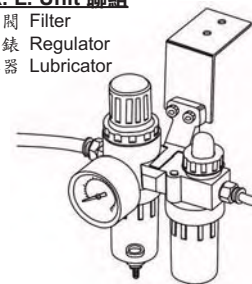
F. R. L. Unit 聯組
